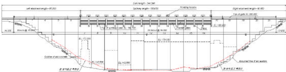
댐체 상류면 부근 바닥표고 측정 현황도
